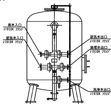
TFRO-TA-〇〇〇-〇〇型 両鏡・自動5方弁
