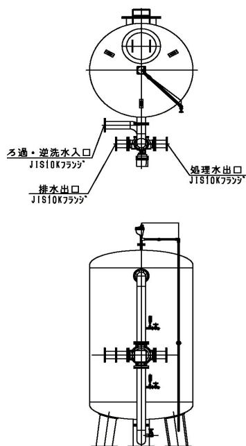
TFRO-JA-〇〇〇-〇〇型 両鏡・自動5方弁
