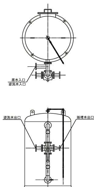
TFBO-JT-〇〇〇-〇〇型 片鏡・手動5方弁
