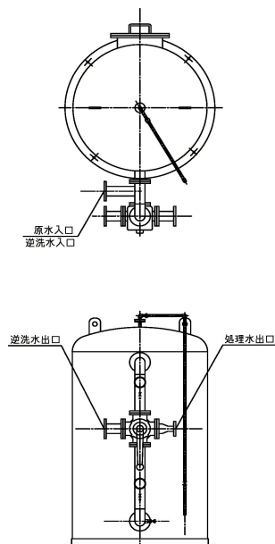
TFBO-JT-000-00型 片鏡・手動5方弁
