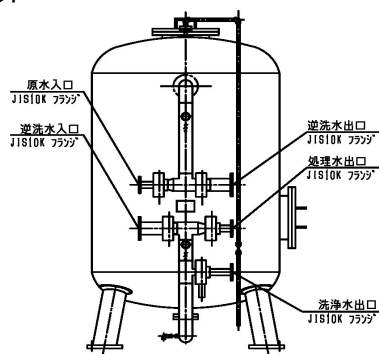
TFRO-TA-000-00型 両鏡・自動5方弁
